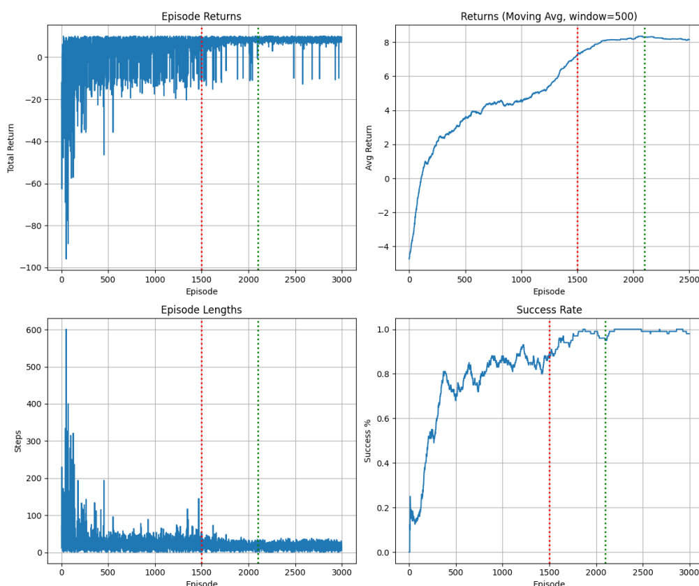
Figura 3: Métricas de entrenamiento en Entorno 1: retornos, media móvil, longitud de episodios y tasa de éxito.
